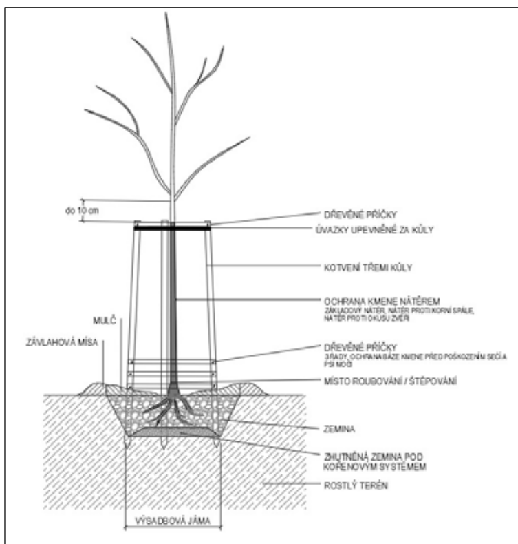
Obrázek: Výsadba stromu – modelový řez
