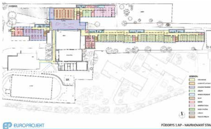
Půdorys 1. nadzemního podlaží po rekonstrukci
