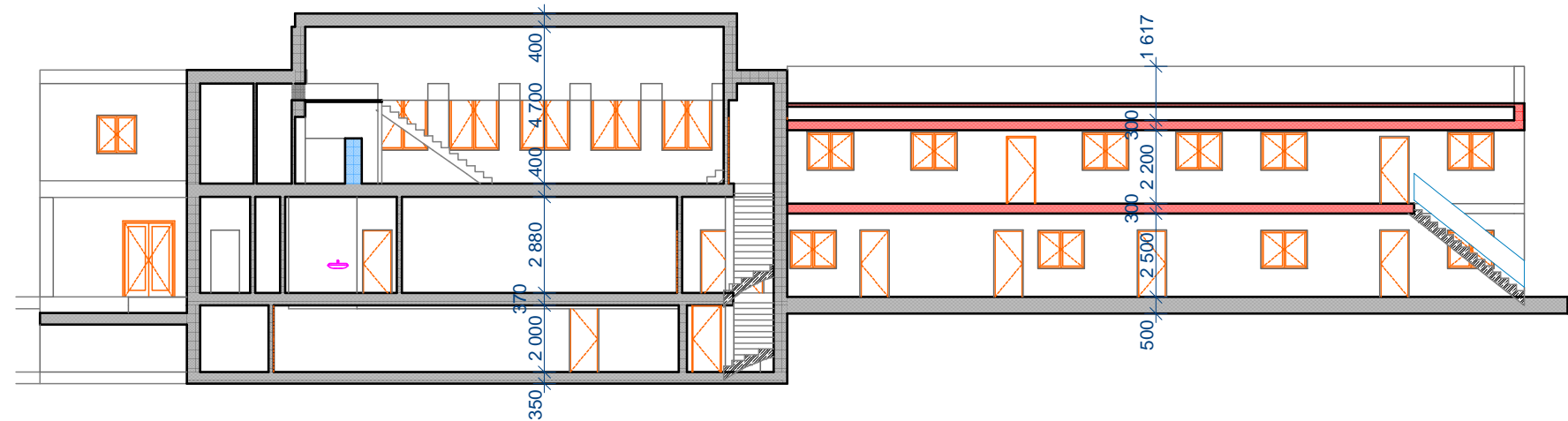
A4 Řez A-A' 1:200
