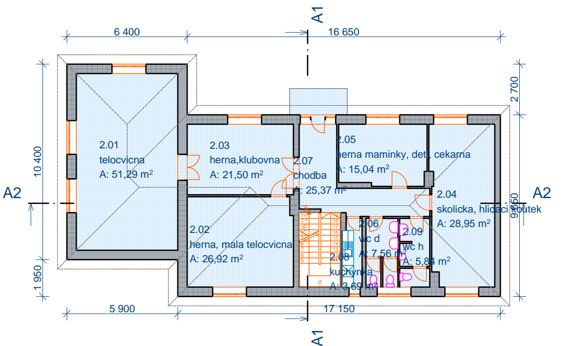
2. 2.NP 1:200
