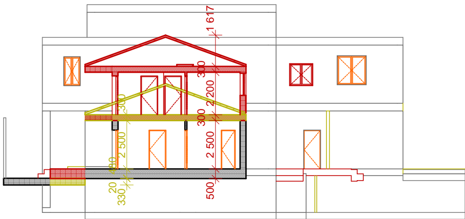
A3 Řez A-A' 1:200
