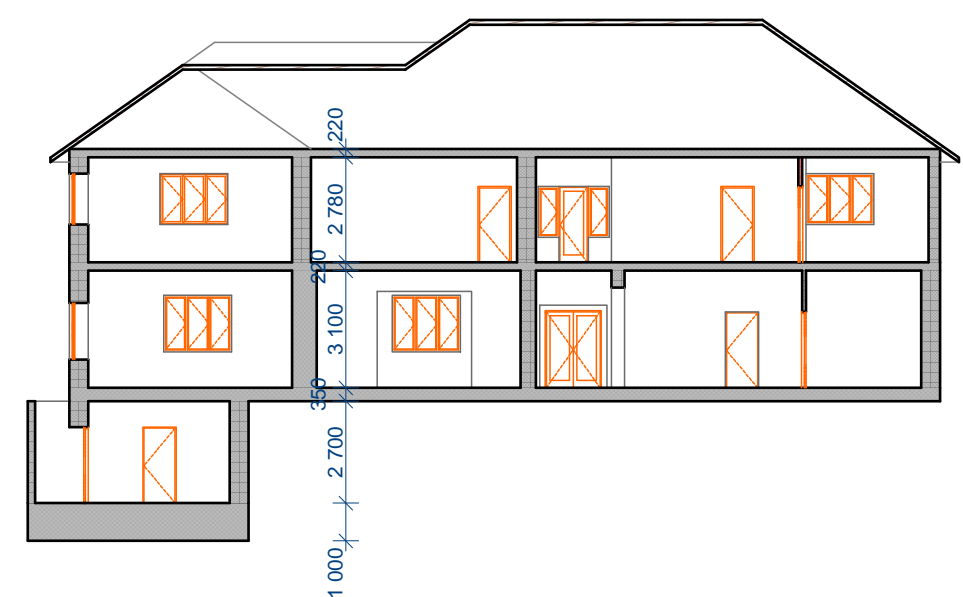
A2 Řez A-A' 1:200
