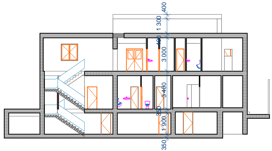
A5 Řez A-A' 1:200
