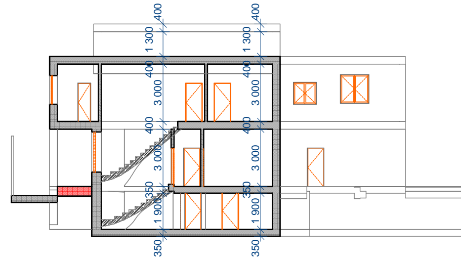
A2 Řez A-A' 1:200
