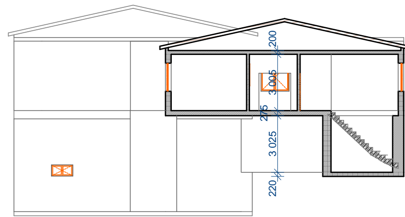
B-B Řez A-A' 1:200
