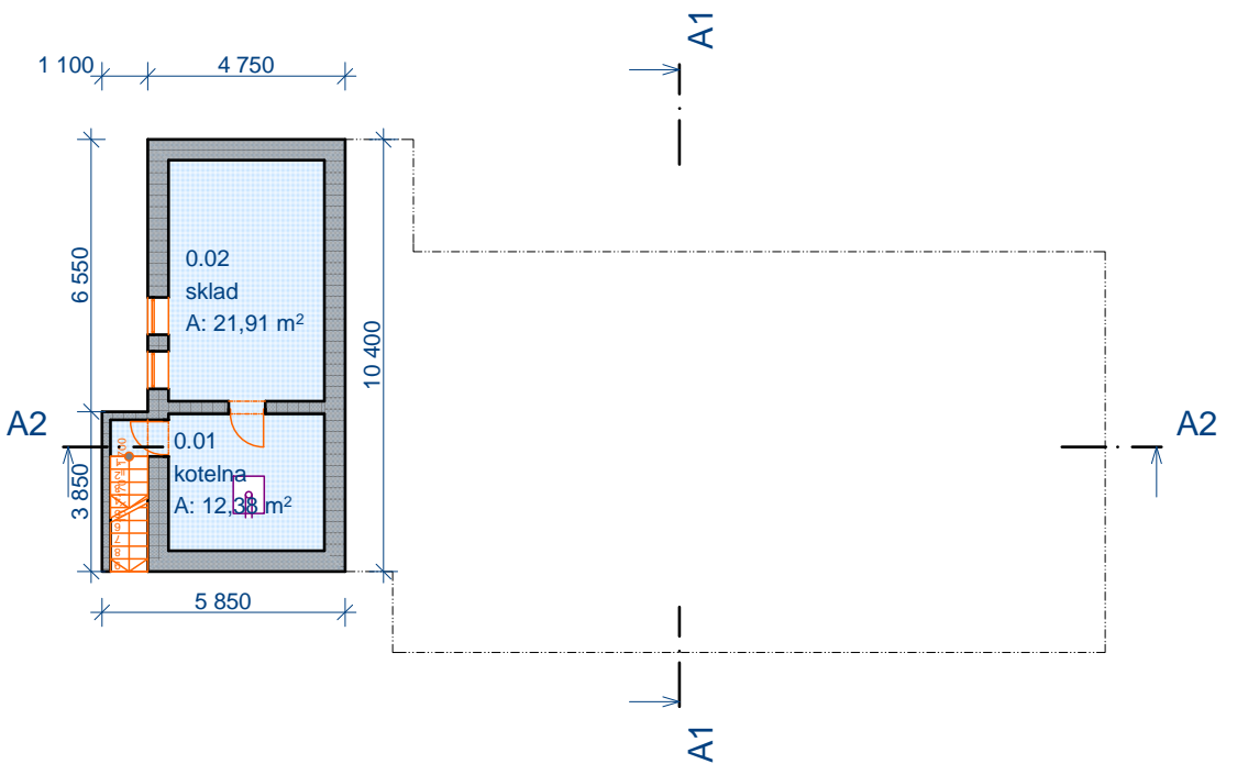
-1. 1.PP 1:200
