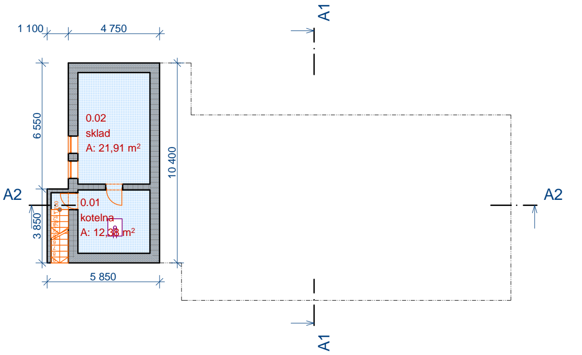
-1. 1.PP 1:200
