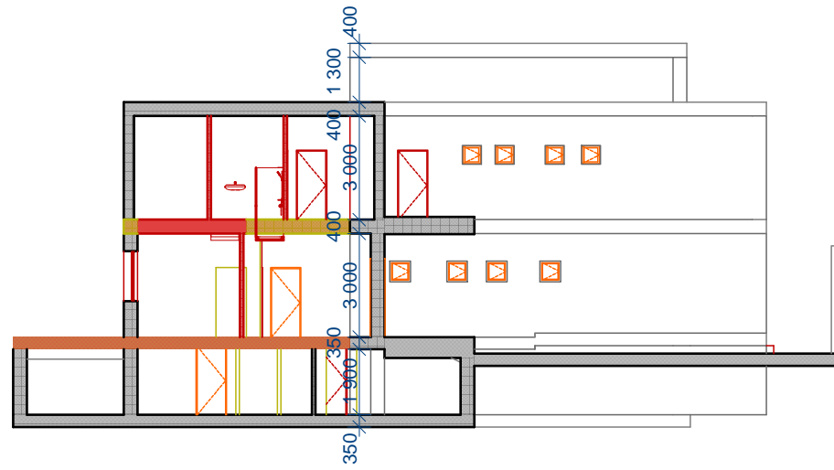
A1 Řez A-A' 1:200
