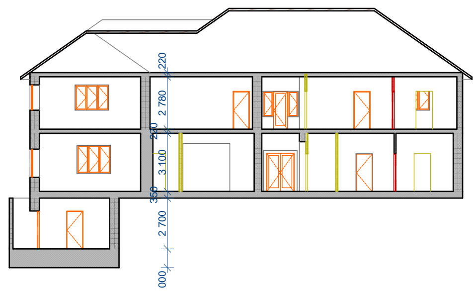
Řez A-A' 1:200
