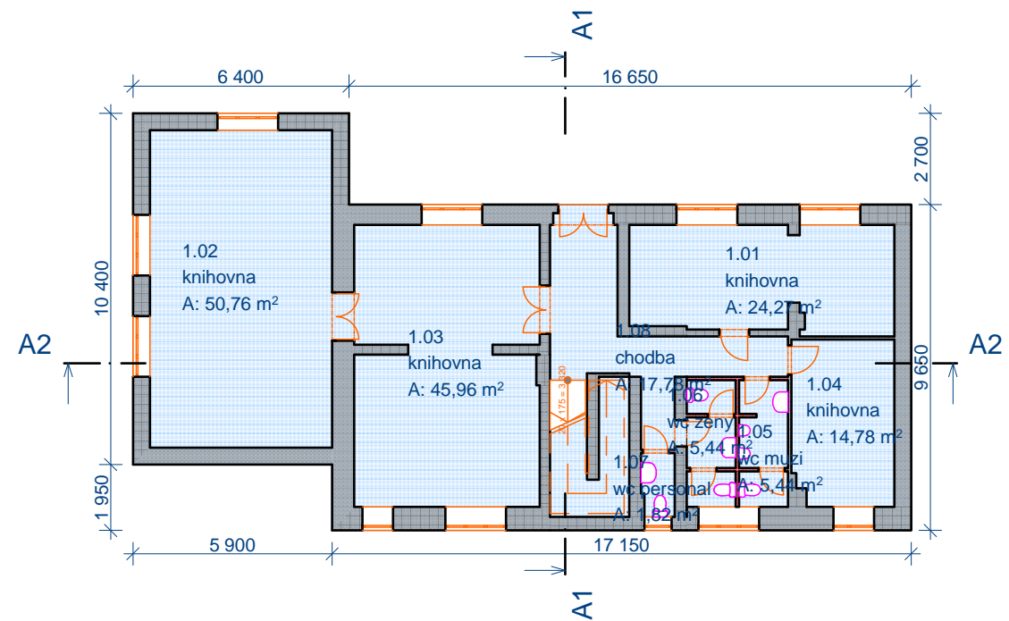
1. 1.NP 1:200
