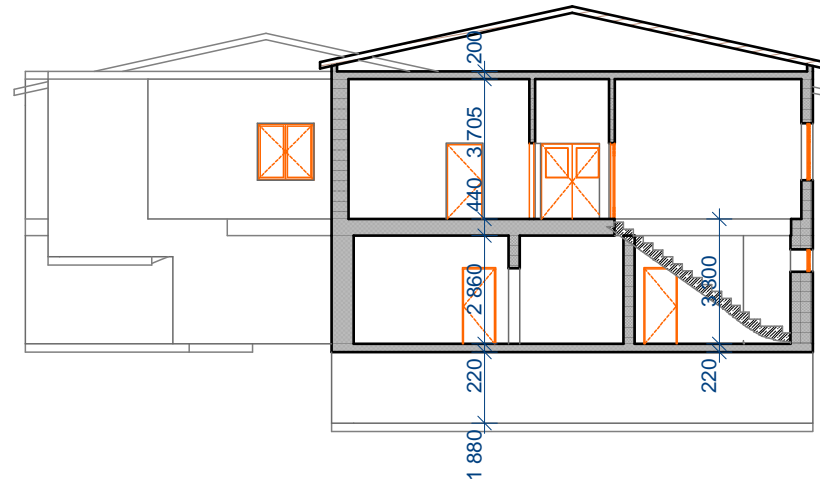
A-A' Řez A-A' 1:200
