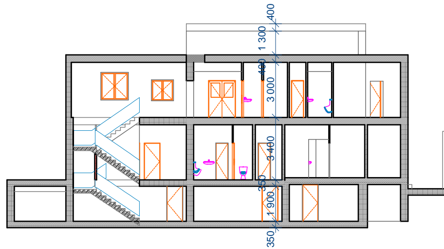
A5 Řez A-A' 1:200
