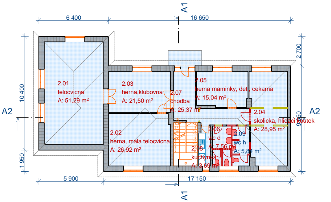
2. 2.NP 1:200
