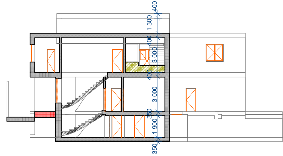
A2 Řez A-A' 1:200
