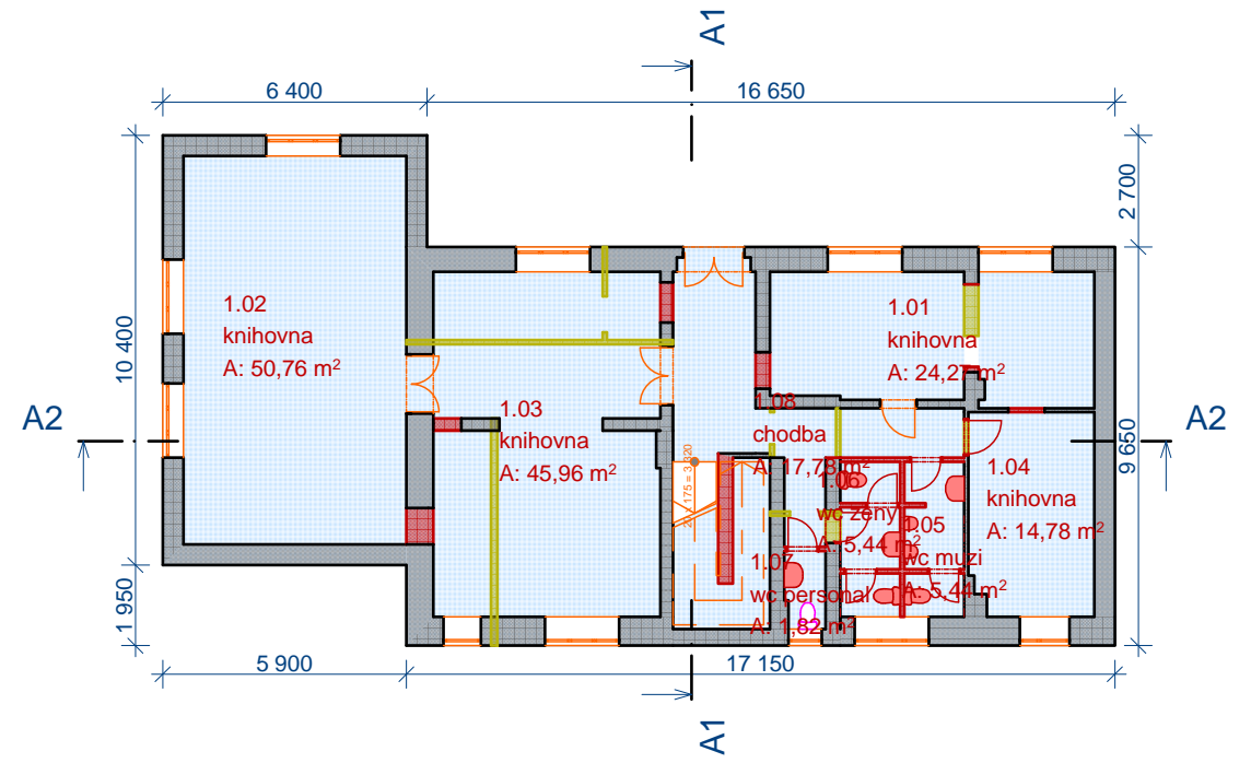
1. 1.NP 1:200
