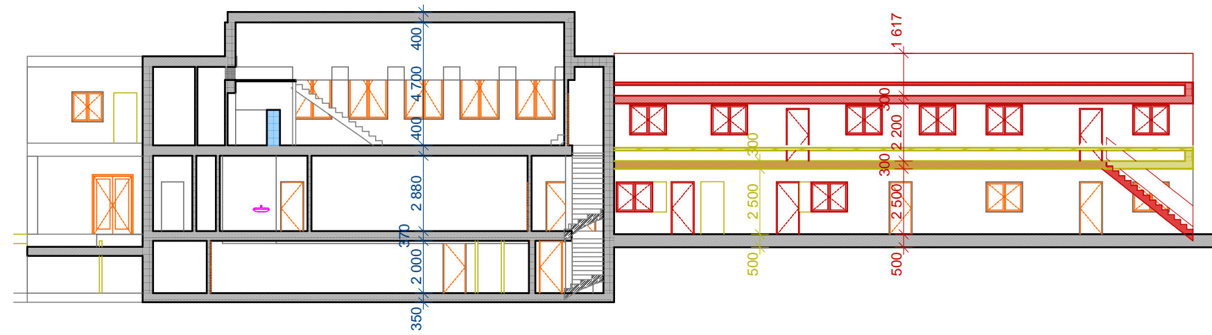
A4 Řez A-A' 1:200
